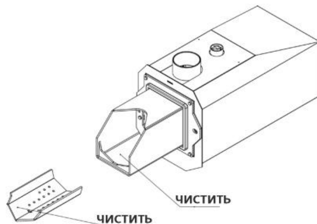
Рис. 06. Чистка горелки
