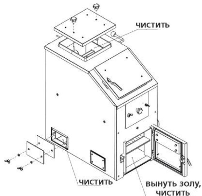
Рис. 05. Чистка котла.
